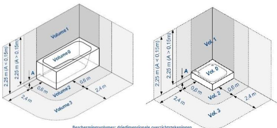
Beschermingsvolumes: driedimensionale overzichtstekeningen
