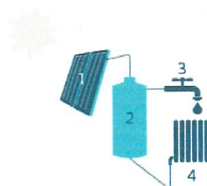
1. Zonnecollector | 2. Opslagvat zonneboiler | 3. Tapwater warm water | 4. Afgiftesysteem voor ruimteverwarming (optioneel)
